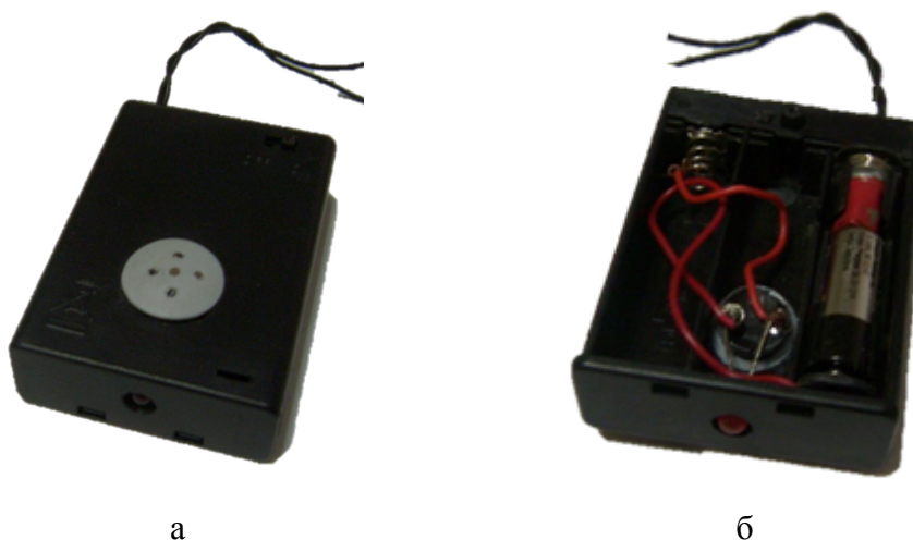
Рисунок 2 – Сигнализатор имитации взрыва (приведения в действие) взрывных устройств: а – внешний вид сигнализатора; б – вид сигнализатора изнутри
