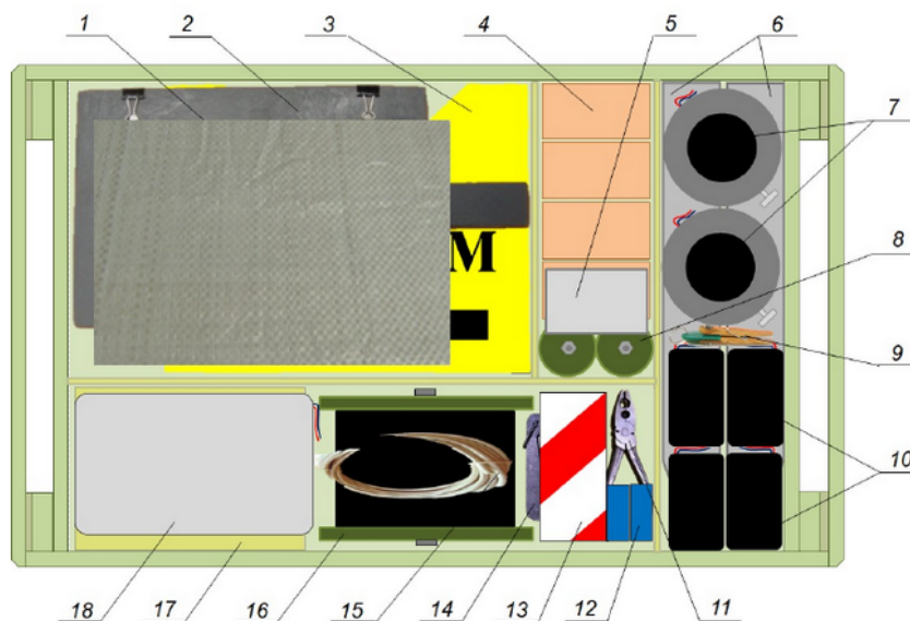
Рисунок 8 – Схема укладки элементов УКМВЗ:
