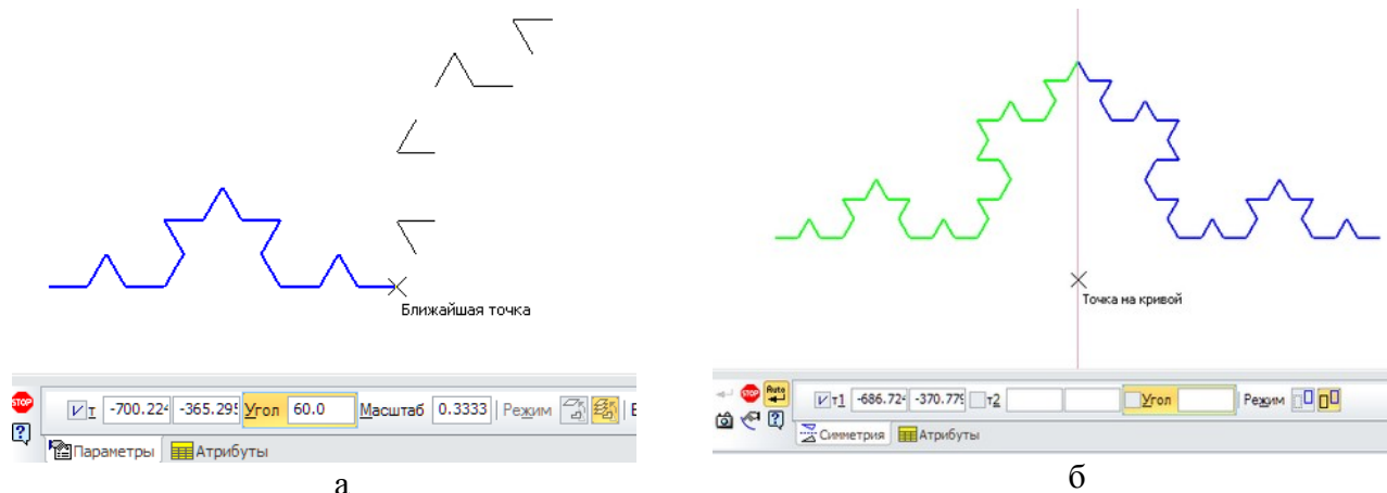
Рисунок 4 – Алгоритм построения третьей итерации кривой Коха с помощью средств векторной графики: а – копирование и вставка под углом 60^\circ ; б – команда Симметрия
