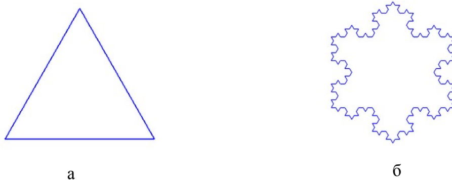
Рисунок 6 – На основе заданного треугольника выполнить 3 итерации снежинки Коха: а – генератор кривой; б – окончательный результат
