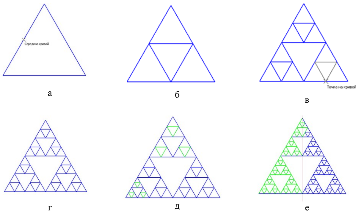
Рисунок 5 – Построение треугольника Серпинского:
