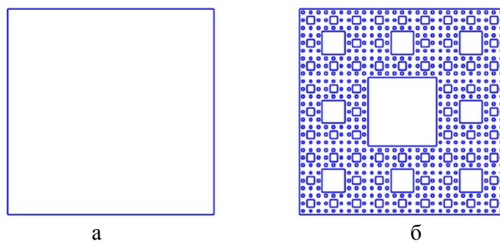
Рисунок 7 – Выполнить первые четыре итерации ковра Серпинского ( r=1/3 ): а – генератор кривой; б – окончательный результат
