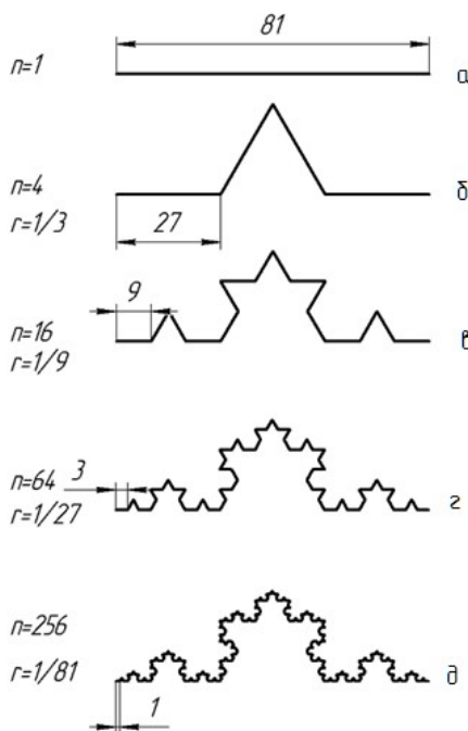
Рисунок 3 – Построение триадной кривой Коха: а – генератор кривой; б – первая итерация; в – вторая итерация; г – третья итерация; д – четвертая итерация
