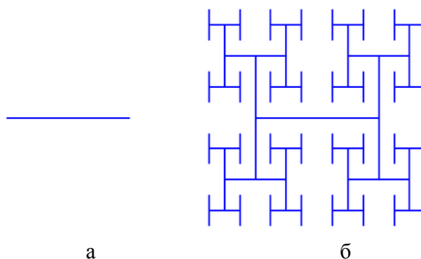
Рисунок 8 – Выполнить первые четыре итерации древа Кейли ( r=1/2 ): а – генератор кривой (отрезок заданной длины); б – окончательный результат
