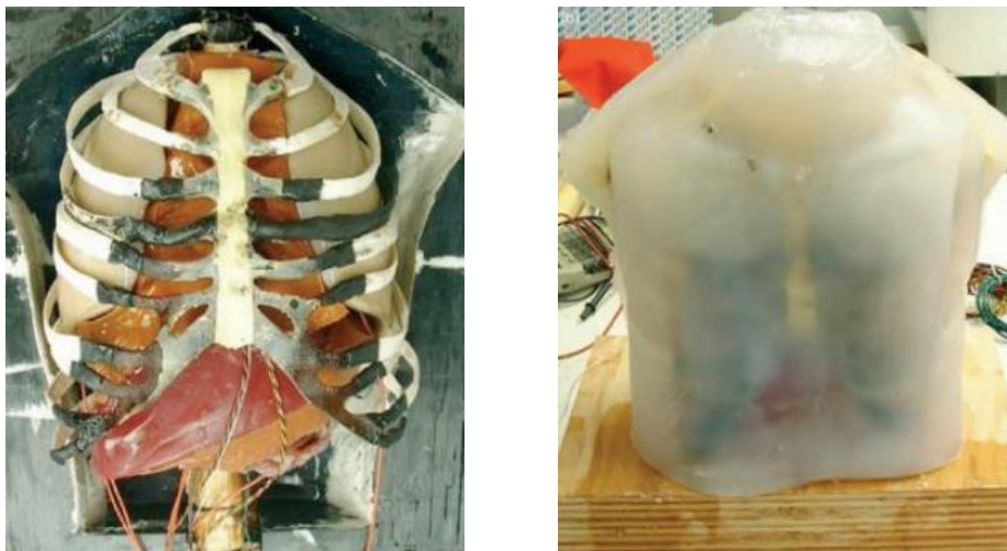
Рисунок 2 – Конструкция антропоморфной модели торса человека с имитацией скелета, внутренних органов, мышц и кожных покровов
