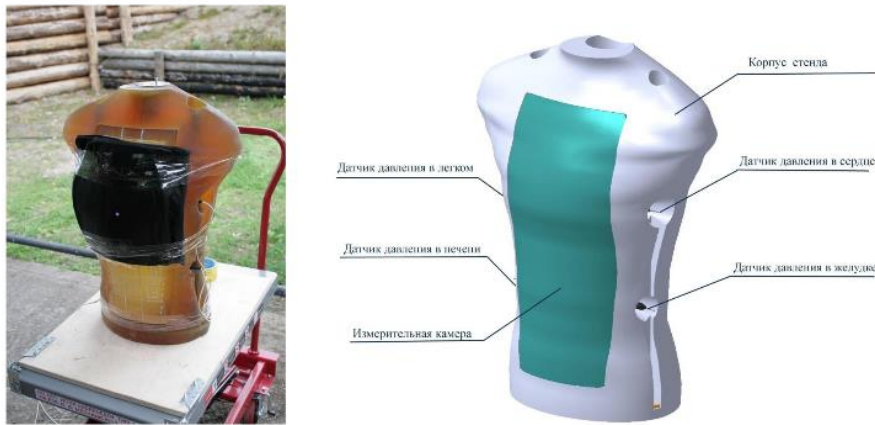
Рисунок 1 – Конструкция антропоморфной модели торса человека со схемой размещения датчиков давления
